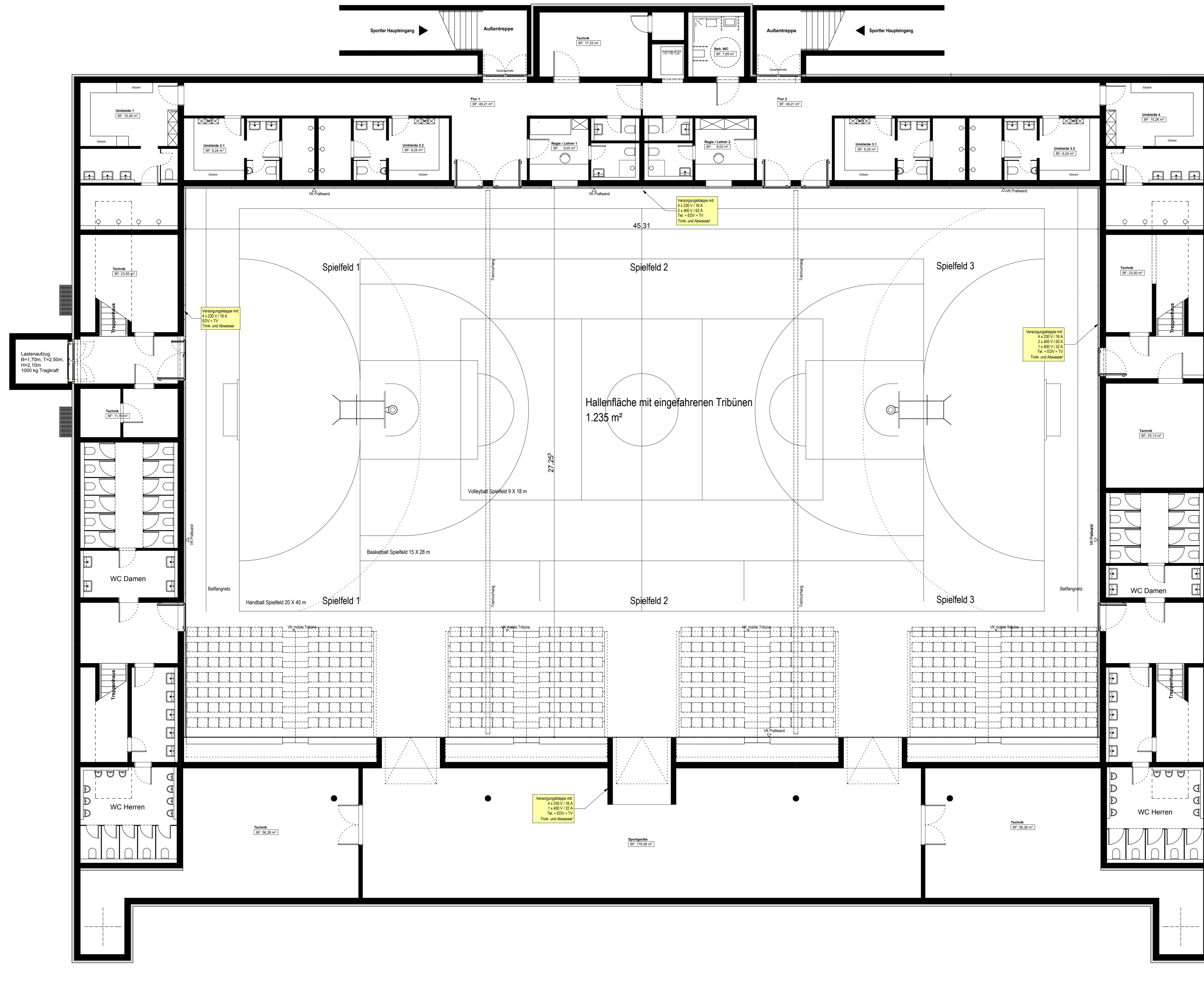
Grundriss Untergeschoss
