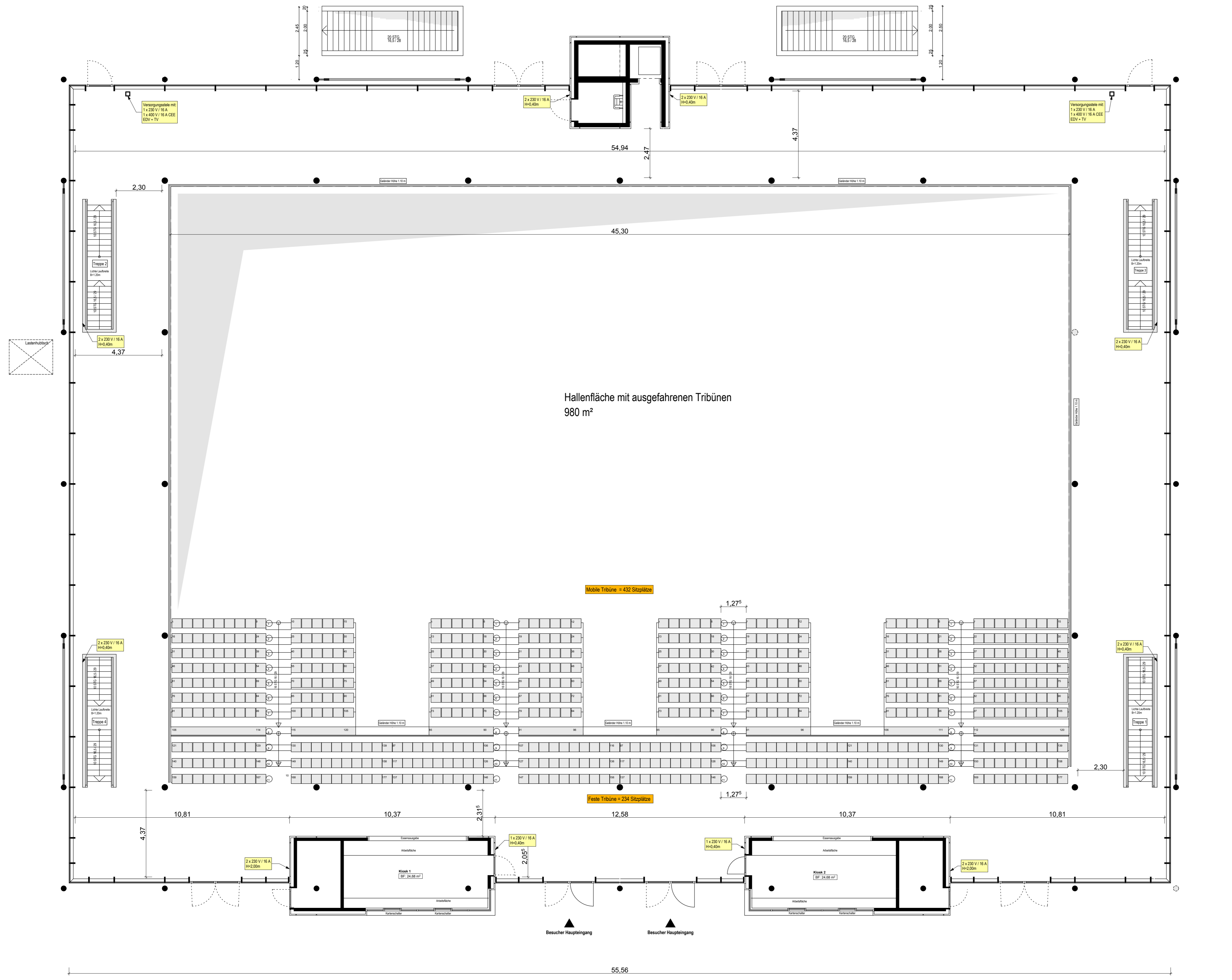
Grundriss Erdgeschoss
